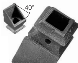
Art. 1491/1 H 50 mm L 30 mm hole for/foro per sezione ∅ 12 x 12 mm
