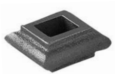
Art. 1390/1 H 17 mm L 38 mm hole for/foro per sezione ∅ 17 x 17 mm
