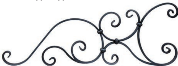
left - sinistro Art. 1281/9 ▧ 20 x 8 mm 310 x 850 mm
