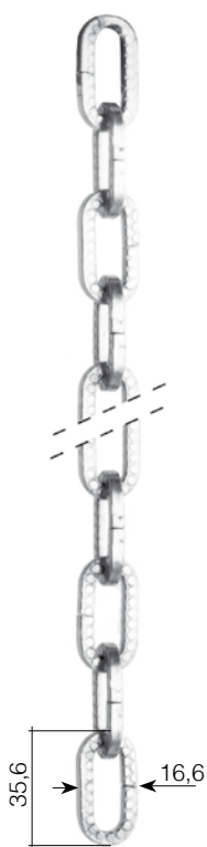
Art. 156/A/12 3,8 x 3,8 mm
