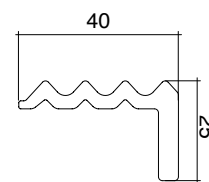
L-Profile Profilo ad elle
