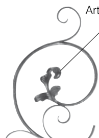
left - sinistro Art. 94/E/3 Ø 12 mm 310 x 540 mm
