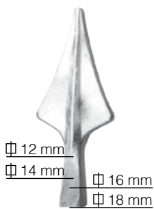
Art. 126/D/1 Ø 12 mm Ø 14 mm Ø 16 mm Ø 18 mm Ø 18 x 18 mm 60 x 155 mm
