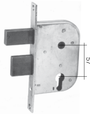
Art. 181/12 Double-lock latch Serratura doppia mandata
